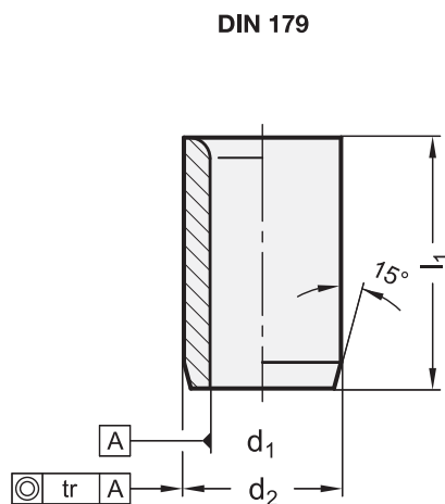
3 Form A Bohrung einseitig gerundet
