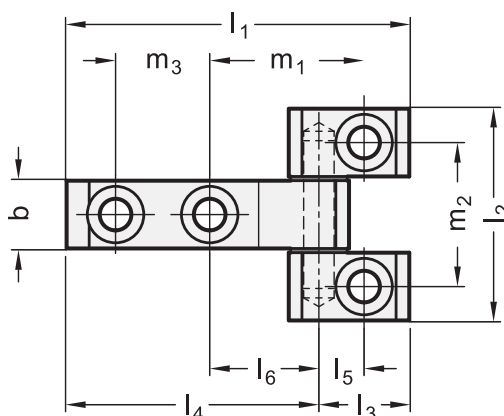
3 Form A Befestigung von der Vorderseite
